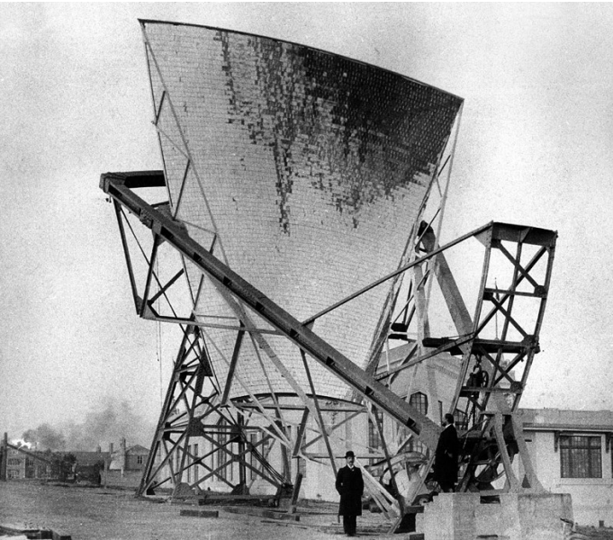
O Pyrheliophero do Padre Himalaya, em 1904, na Exposição Universal de St. Louis, EUA Coleção particular de Jacinto Rodrigues
